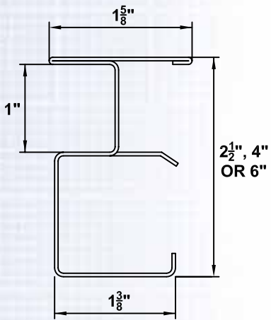
CT STUD
