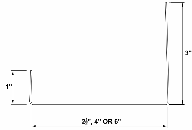
JAMB TRACK
